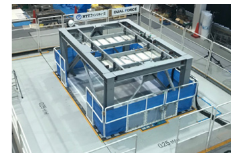
「DUAL FORCE」を使用した実大実験風景
