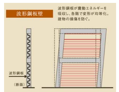
波形鋼板壁
